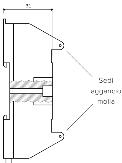
Vista laterale
